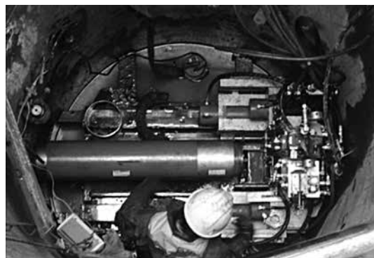
写真-1 ケーシング立坑での施工状況 1)
