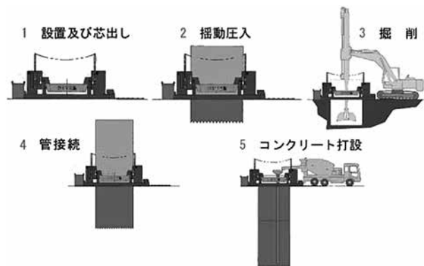
図-1 鋼製ケーシング施工手順 2)
